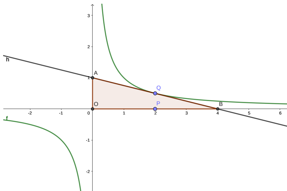
Figura 11: Não importa que ponto na tangente escolhemos, a área do triângulo é sempre 2c .
