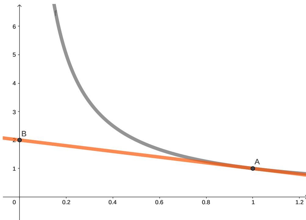
Figura 12: À medida que o ponto A se move pra direita, o ponto B desce em direção à origem. O problema está perguntando — quão rápido B está descendo quando A passa pelo ponto x = 1 ?
