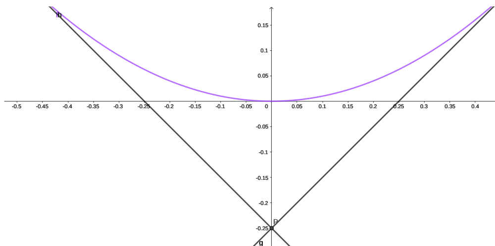
Figura 10: O ponto (0, -1/4) é a interseção entre as tangentes à curva x^2 que são perpendiculares.
